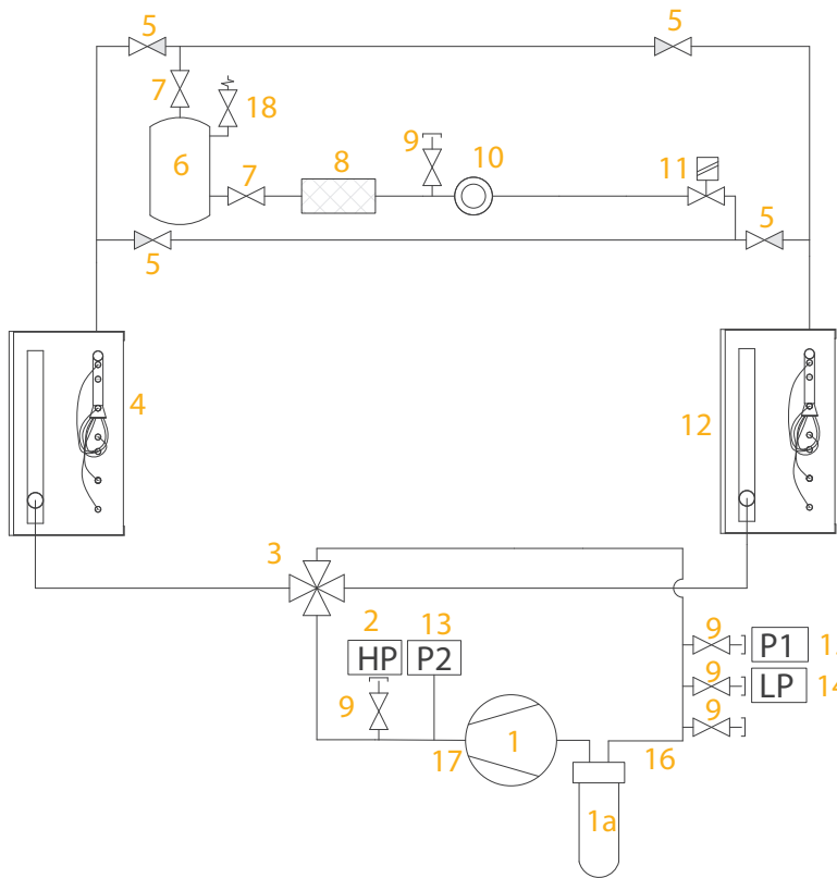
Chladicí systém s tepelným čerpadlem
